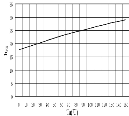
h_{FE} - T_a
