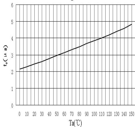
t_s - T_a
