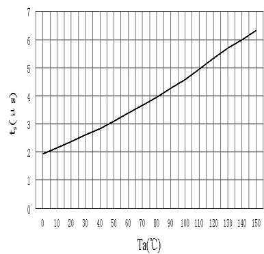
t_s-T_a
