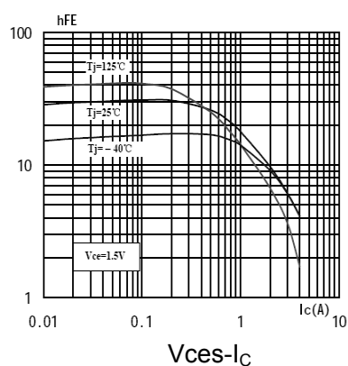
h_{FE}-I_C
