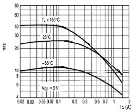
h_{FE} - I_C
