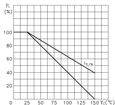
P_C-T_C
