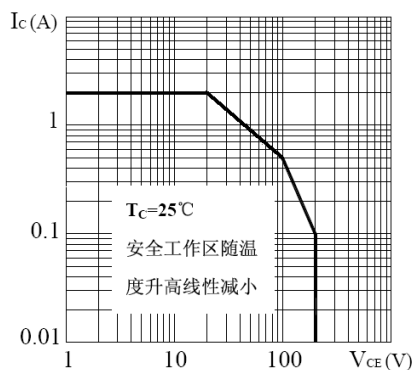
SOA(DC)
