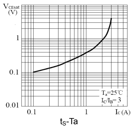
V_{CES}-I_C
