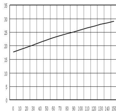
h_{FE}-T_a
