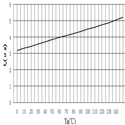
t_s-T_a
