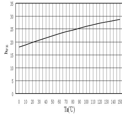
h_{FE}-T_a
