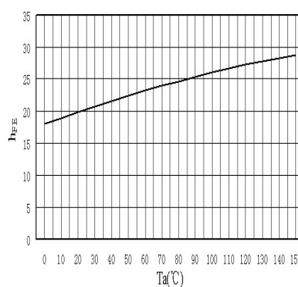
h_{FE}-T_a
