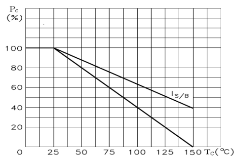
P_C-T_C
