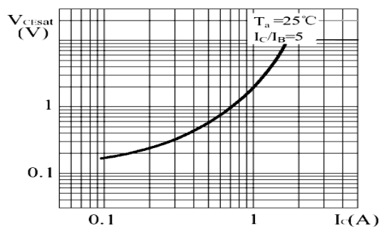
V_{ces}-I_C
