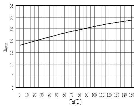
h_{FE}-T_a
