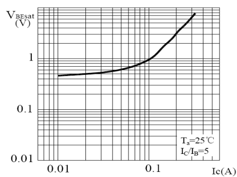
V_{BES}-I_C
