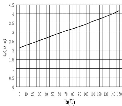
t_s-T_a
