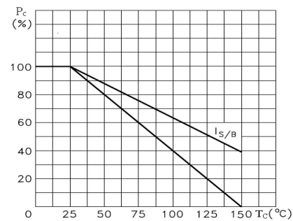
P_C-T_C
