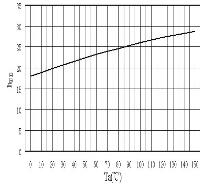
h_{FE} - T_a
