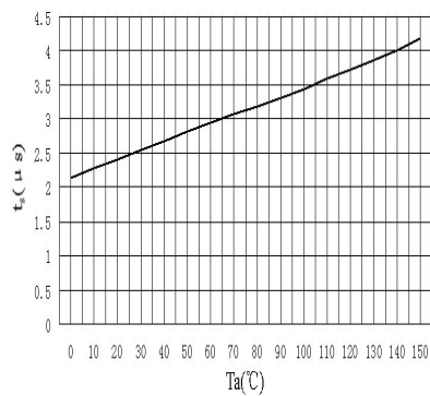
t_s - T_a
