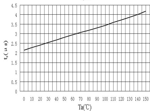
t_s-T_a
