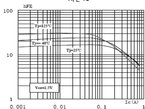
h_{FE}-I_C
