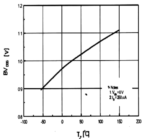
BV_{DSS} - T_J
