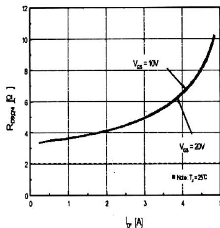
R_{DS(on)} - I_D
